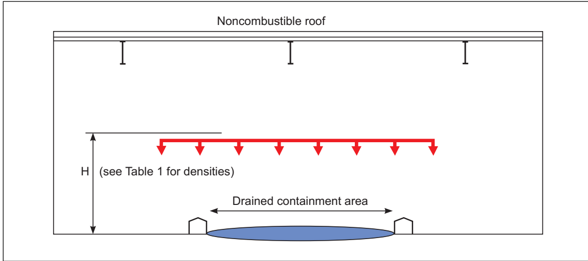
Fig. 2.4.4.2.2(B). Local sprinkler option
