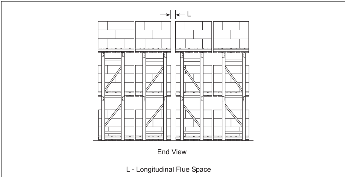
Fig. A-8. Multiple-row rack
