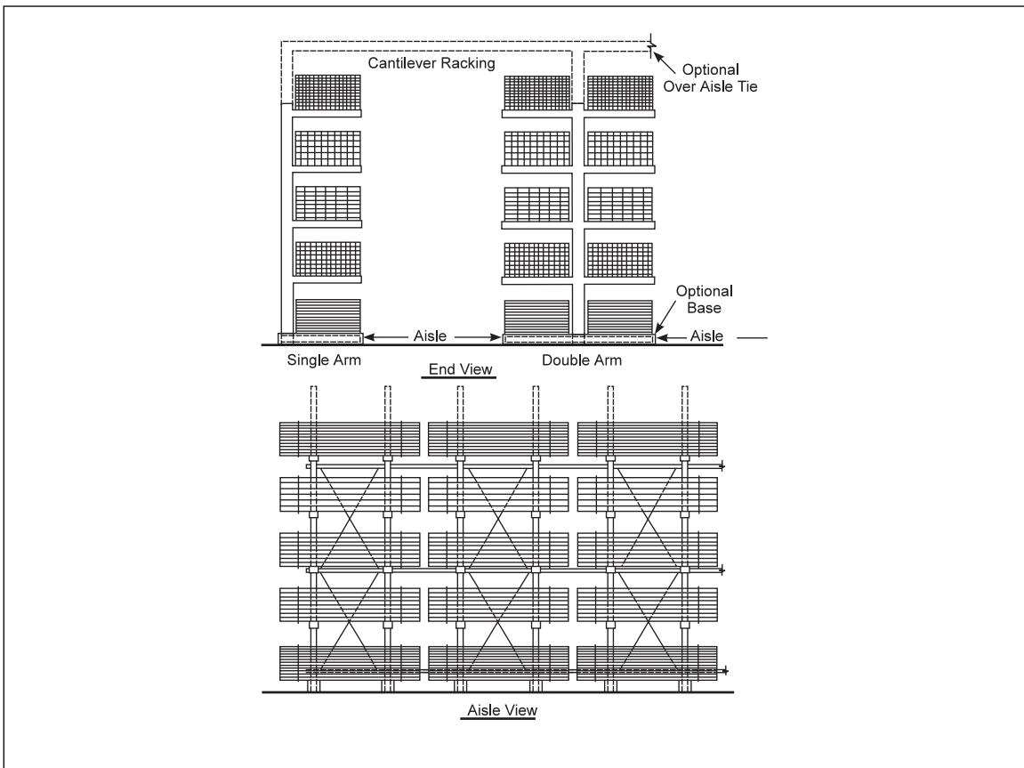
Fig. A-12. Cantilever rack
